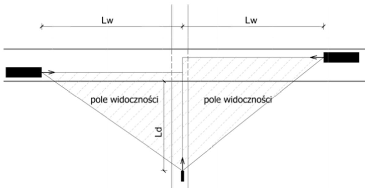
Rys. 4.1. Zasada wyznaczania pola widoczności przy zbliżaniu się rowerem do przejazdu dla rowerów
